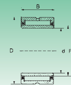
NKI ( d \geq 9 mm) NKIS ( d \geq 8 mm) NA 49/48 NA 69 ( d \leq 30 mm)
