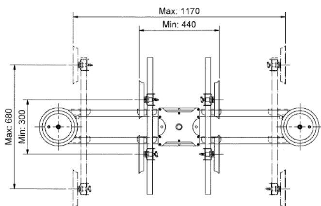
Uiterste standen optie kastoppak Scale ( 1 : 10 )
