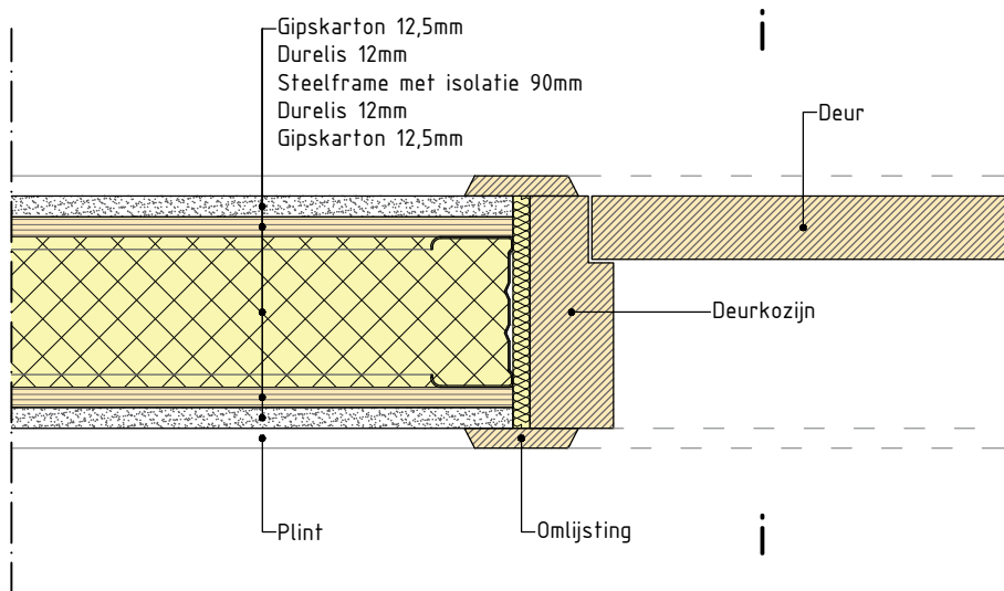
8.1 Binnendeur met omlijsting
