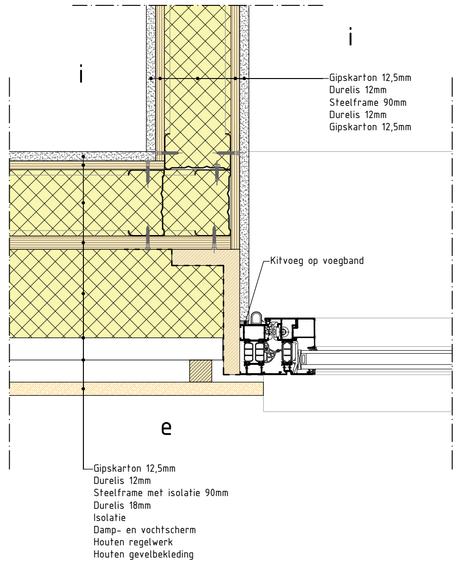
6.9.4 Met houten gevelbekleding 6.9.2 Raamaansluiting - tegen binnenwand
