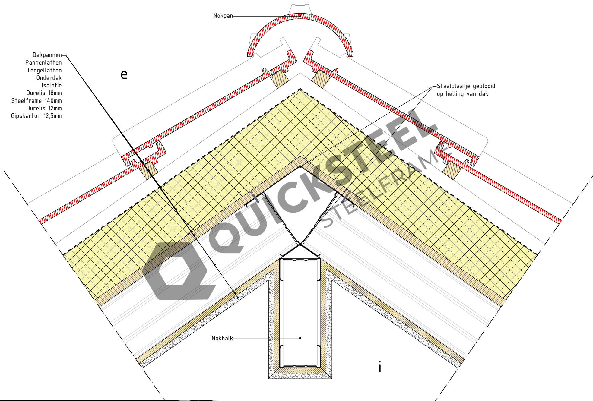
5.9.1 Opbouw hellend dak - daknok met nokbalk
