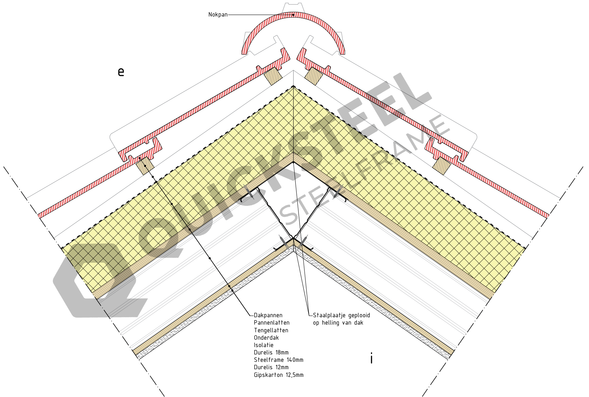
5.9 Opbouw hellend dak - daknok
