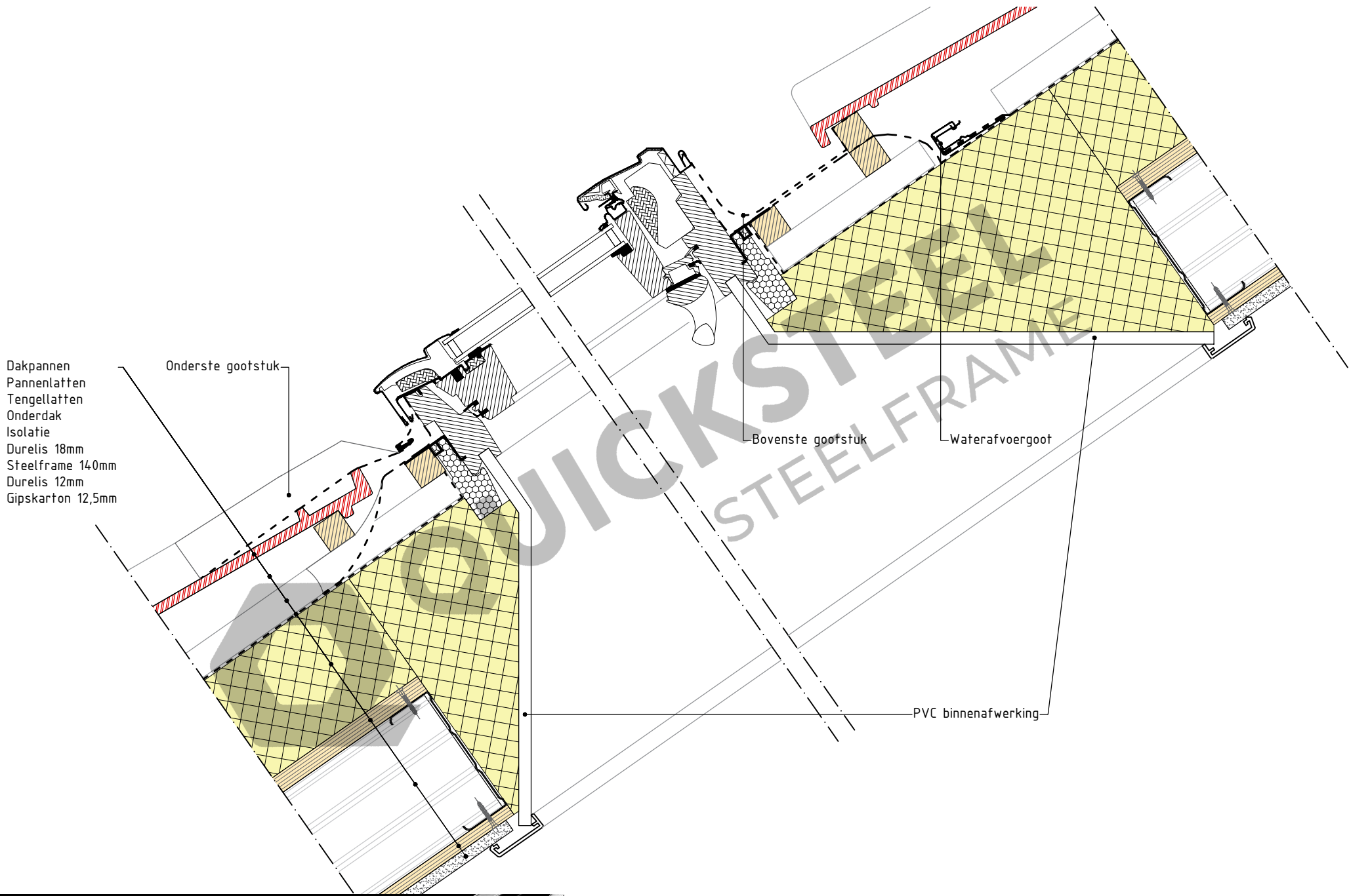
5.8 Opbouw hellend dak - dakraam
