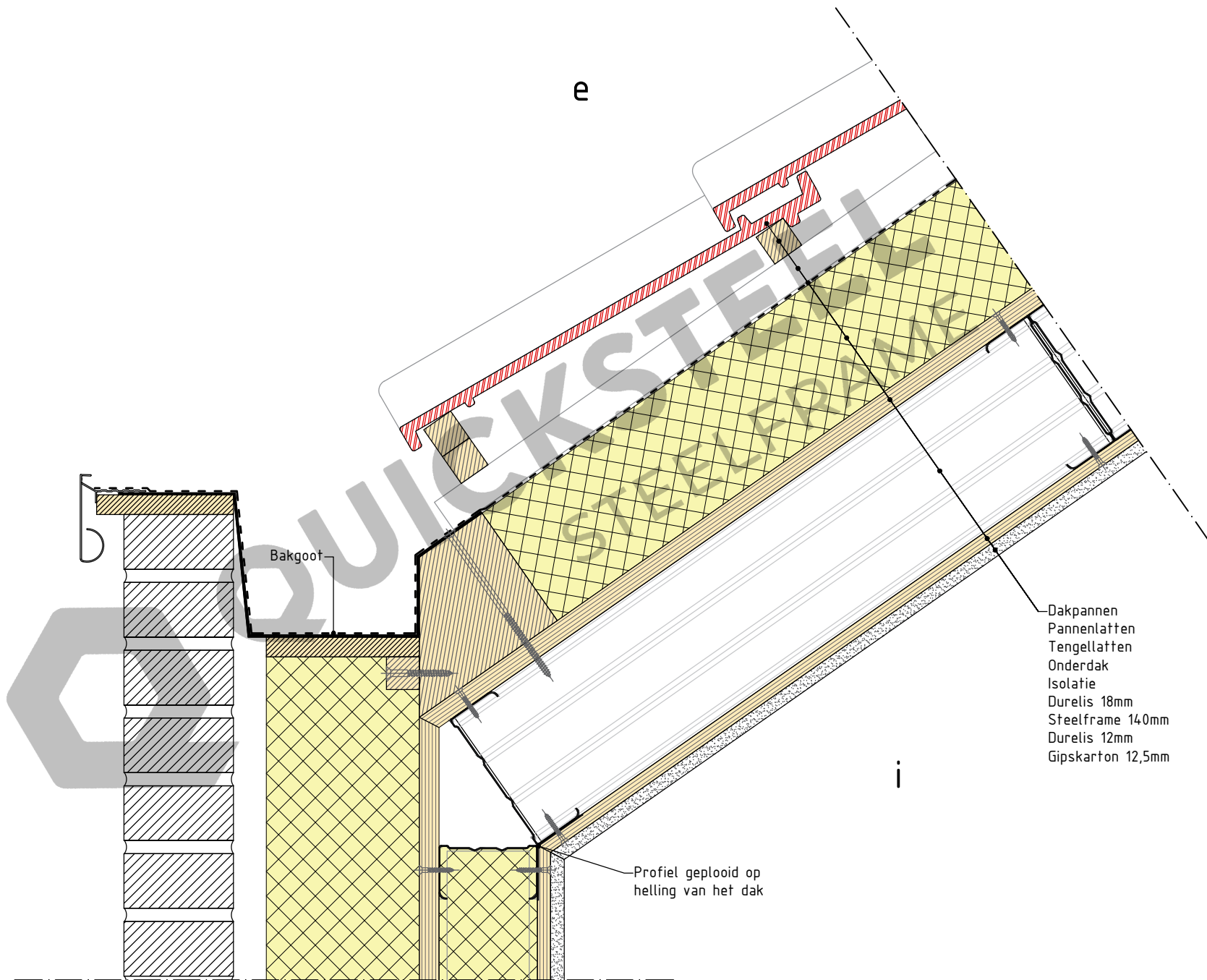
5.5 Opbouw hellend dak - met bakgoot achter de muur
