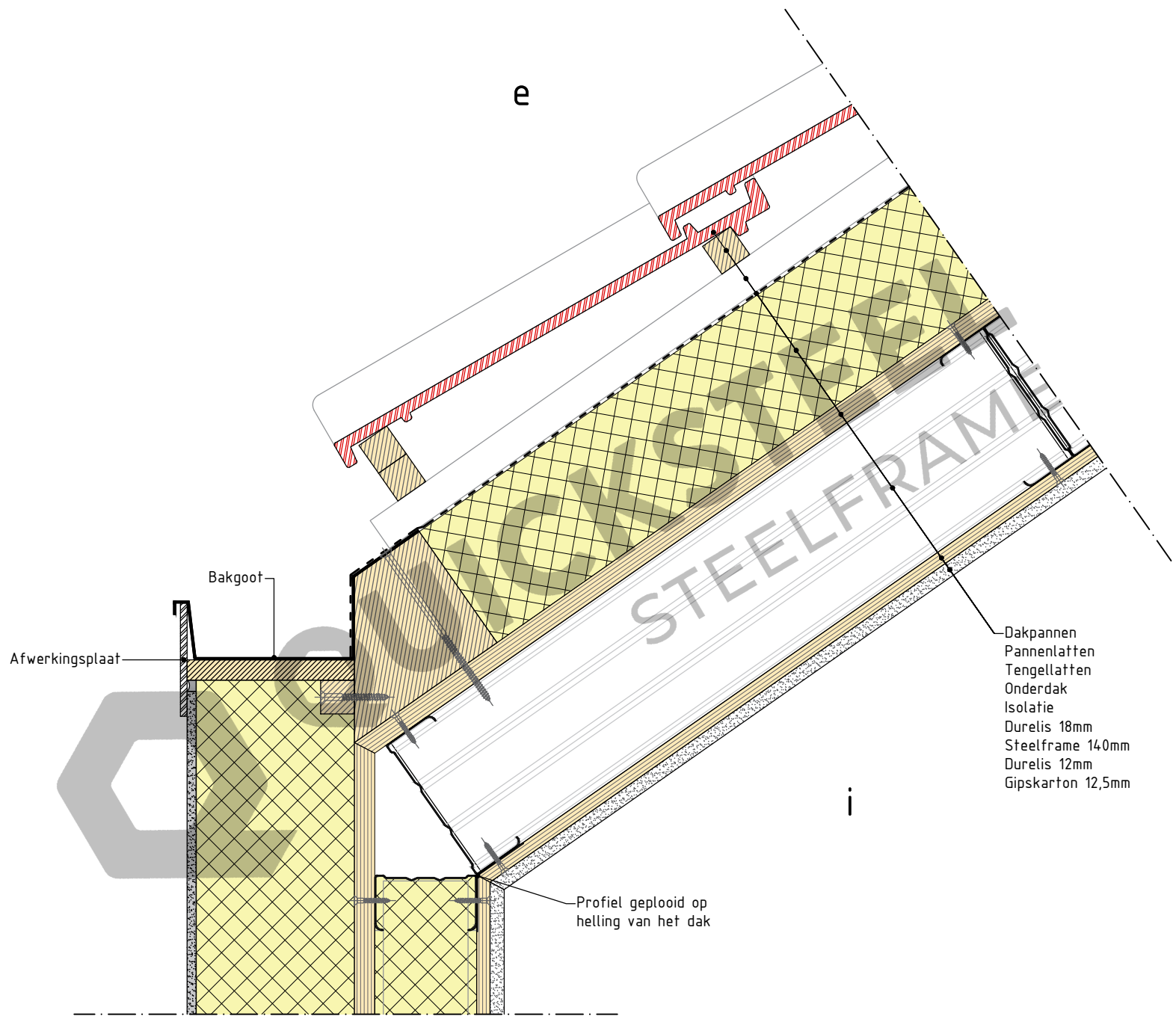
5.3 Opbouw hellend dak - met bakgoot
