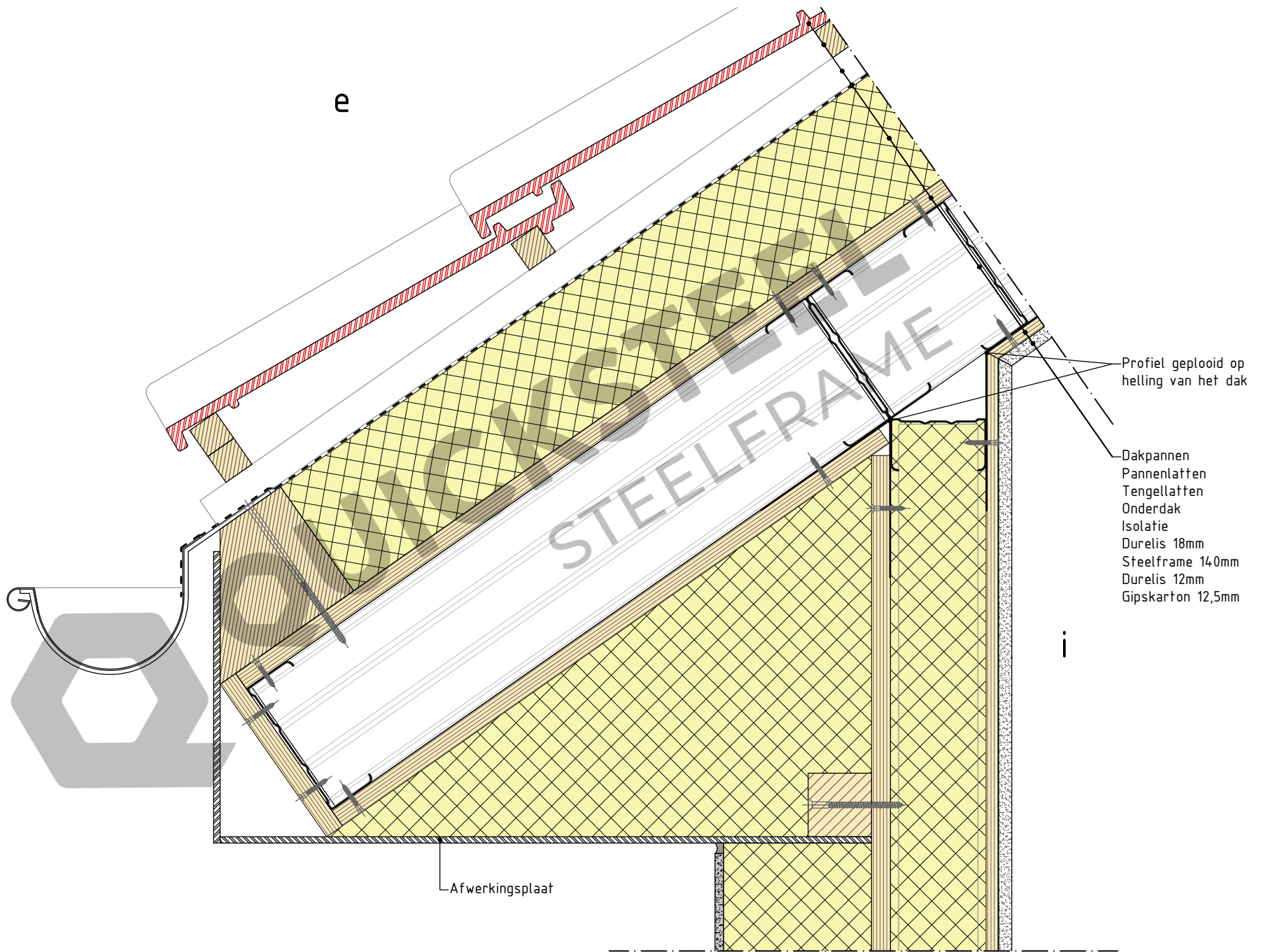
5.2 Opbouw hellend dak - met hanggoot in oversteek
