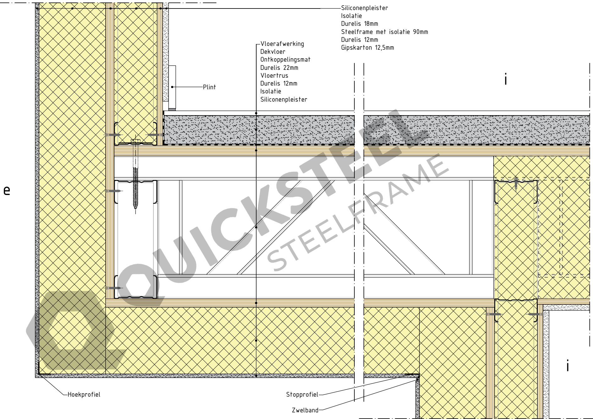
4.3 Opbouw plat dak met oversteek - type 1
