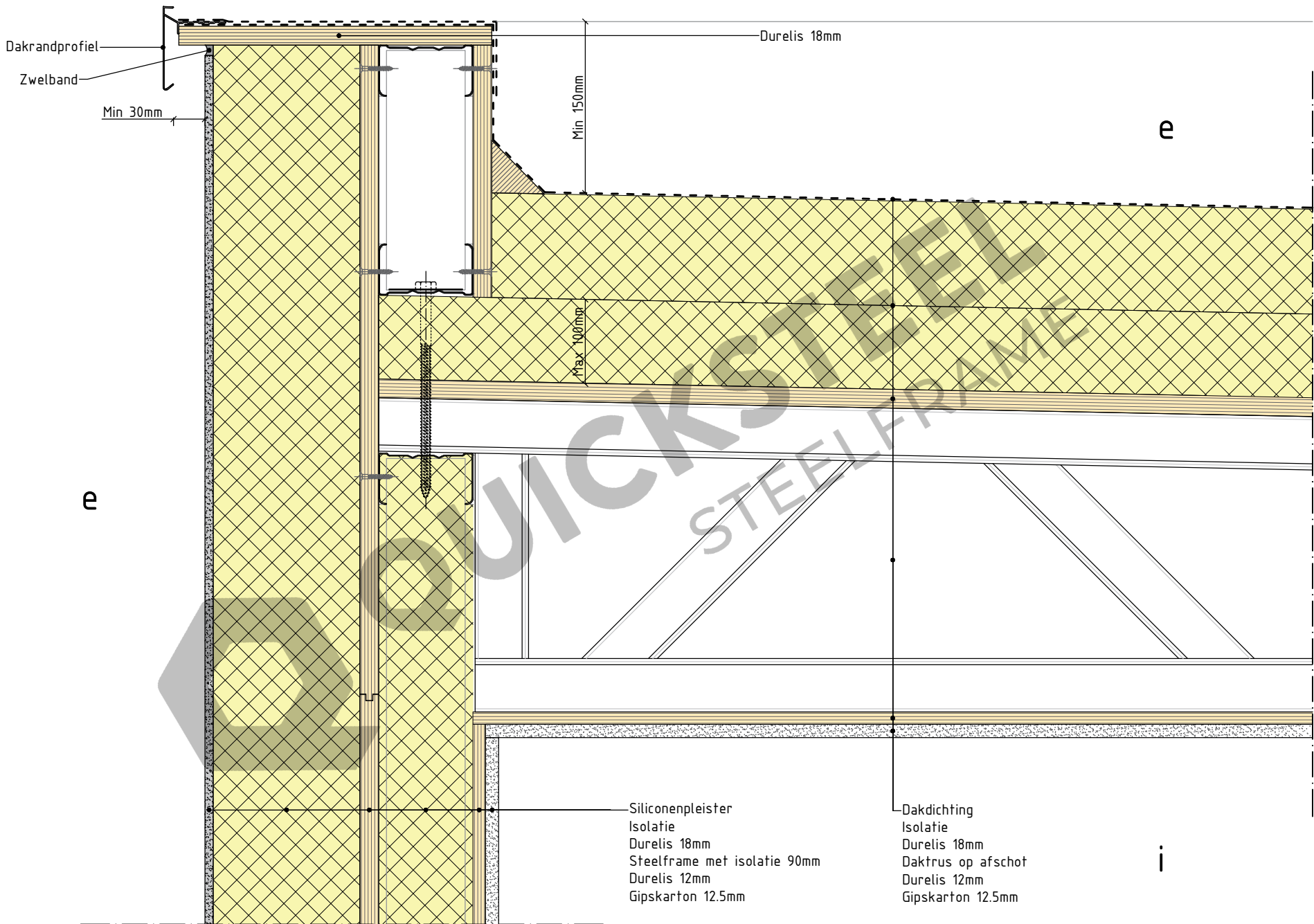
4.2 Opbouw plat dak - met thermische onderbreking
