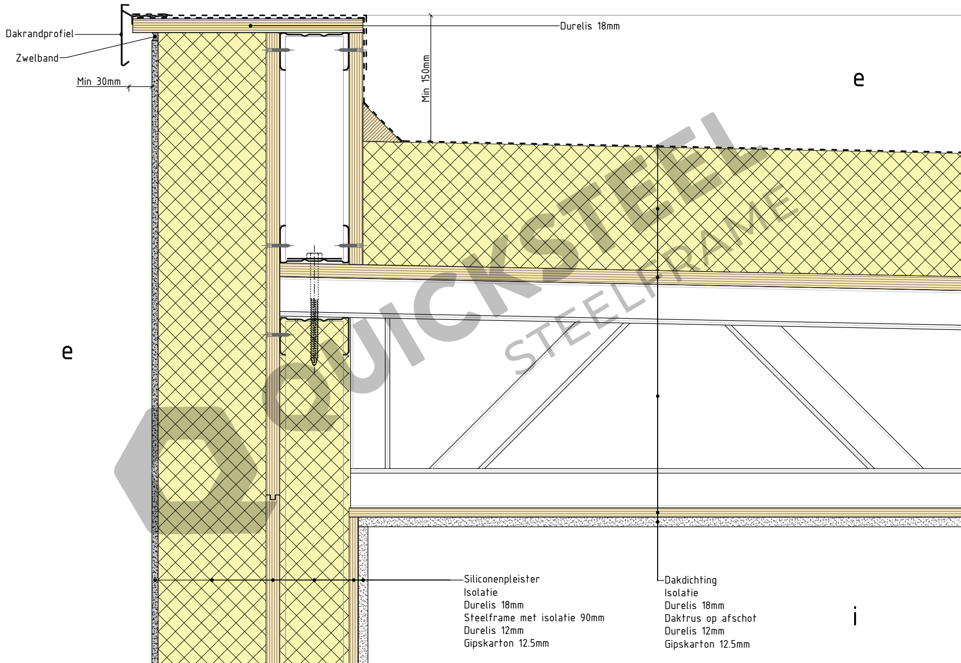
4.1 Opbouw plat dak - zonder thermische onderbreking
