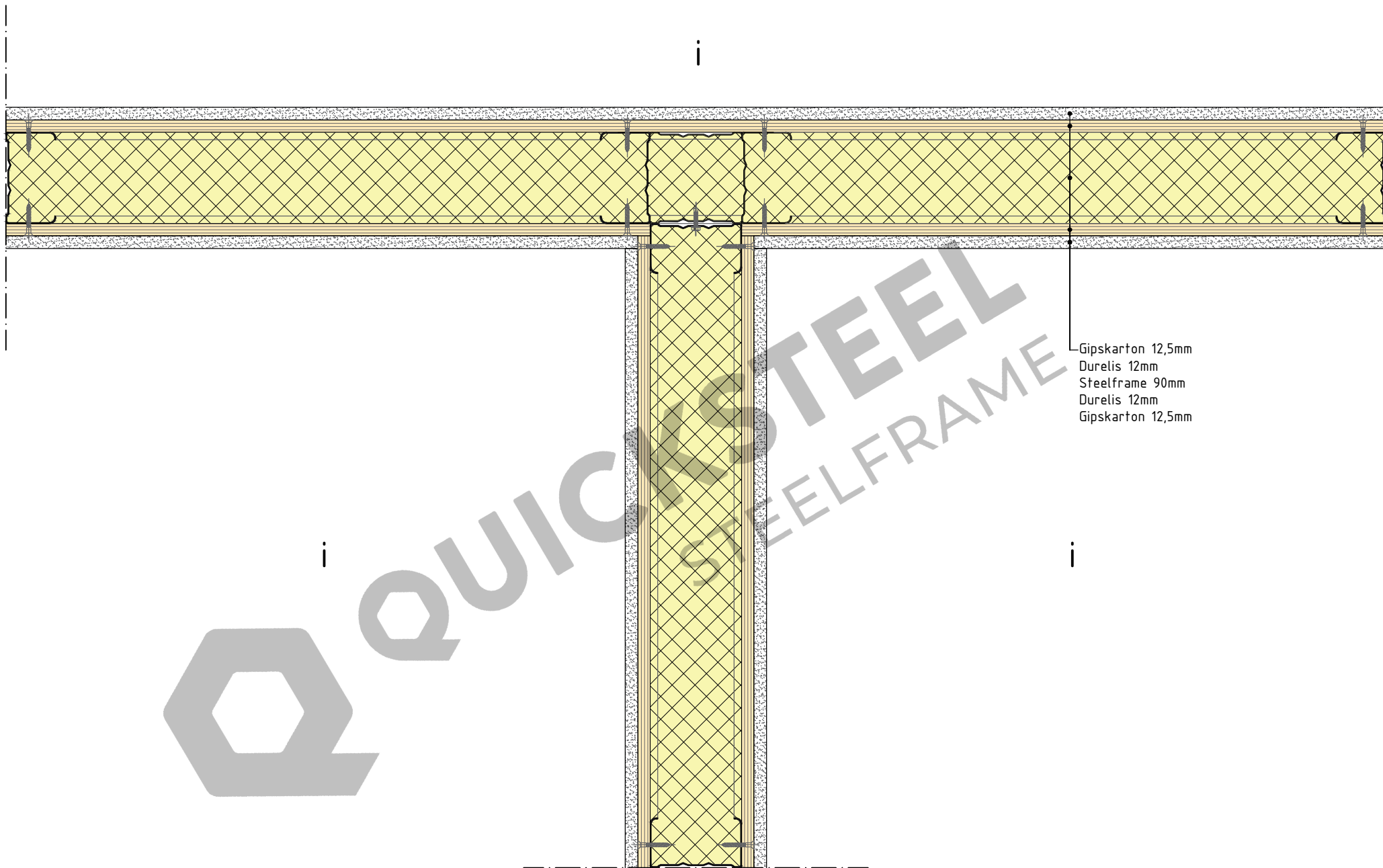
2.1 Verbinding binnenwanden - type 1
