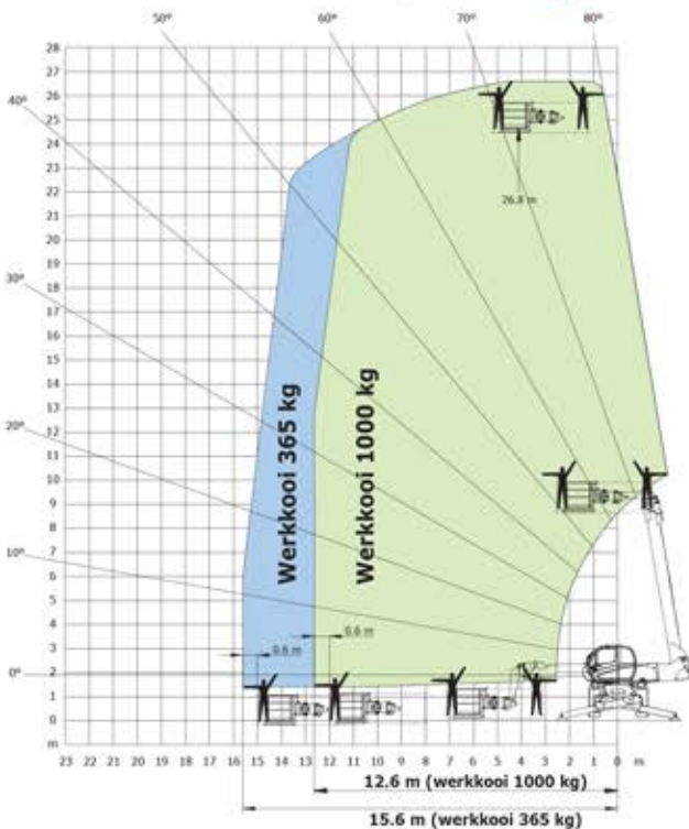
Rotatie op stempels met werkkooi 365/1000 kg
