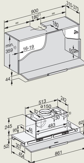
DAS 8930
