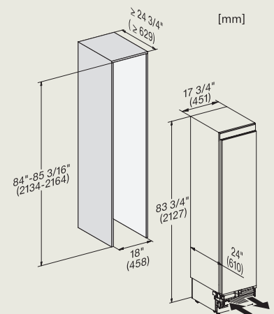
F 2413 Vi
