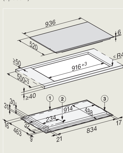
KM 7999 FL (opbouw)
