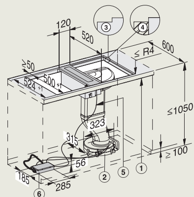
CSDA 7001 FL (vlakbouw)
