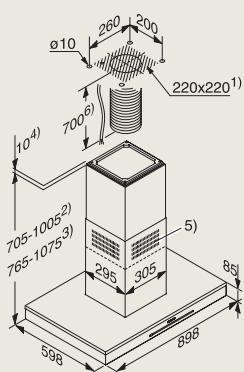
DA 6698 D eilanddampkap
