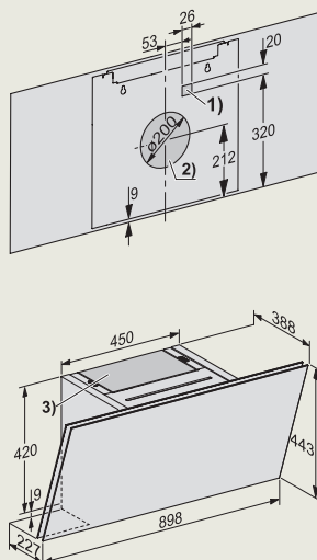
DAH 2960 Escala Hoofdrijke wanddampkap
