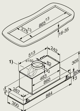
DA 2698 inbouwgroep
