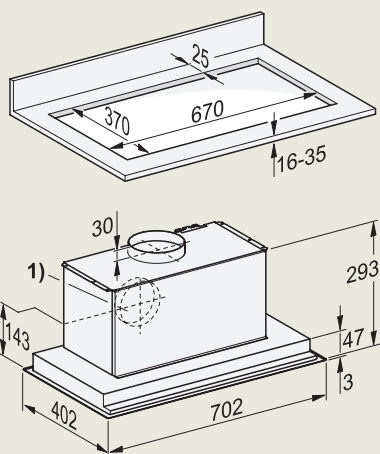
DA 2578 inbouwgroep
