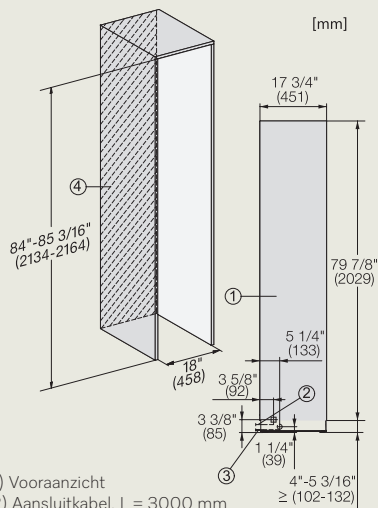
F 2413 Vi - aansluitingen
