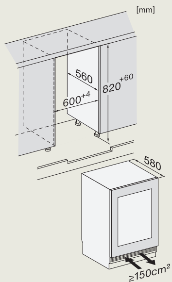
KWTUS 7074 F, KWTUS 7096 E
