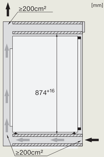
FNS 7140 C
