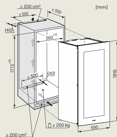
KWT 6722 iGS-1
