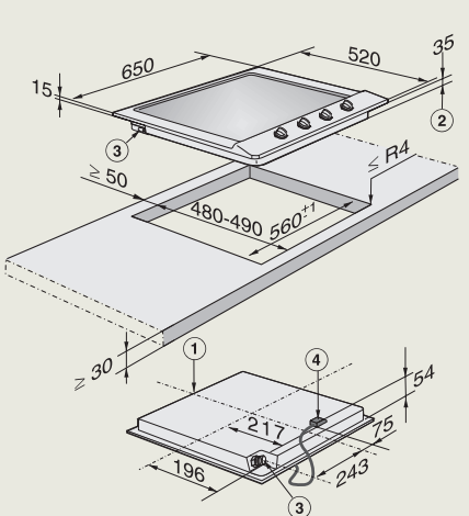
KM 2010
