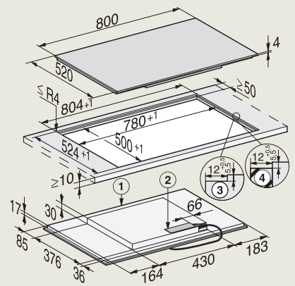
KM 7474 FL (vlakbouw)
