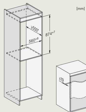
K 7125 E, K 7126 E, K 7127 D
