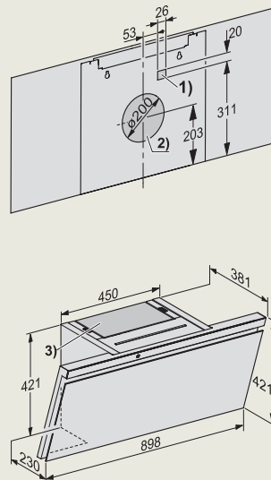
DAH 4970 Sienna, DAH 4980 Hoofdrijke wanddampkap
