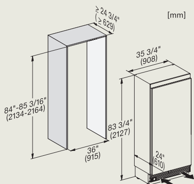
K 2902 Vi
