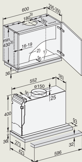
DAS 2620, DAS 4620
