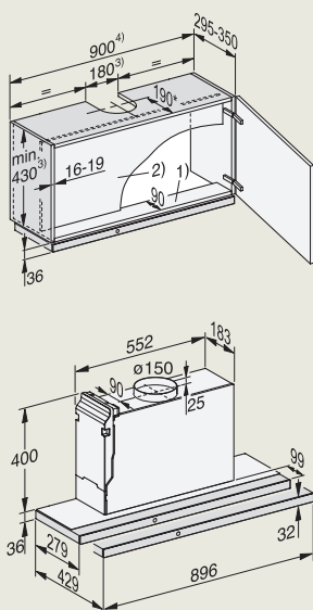
DAS 4930
