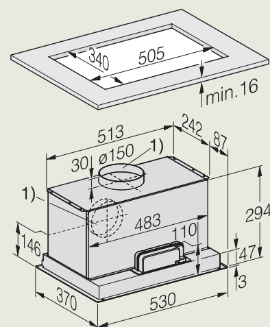
DAE 1530 inbouwgroep
