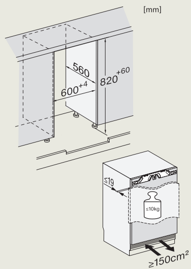
K 7216 E
