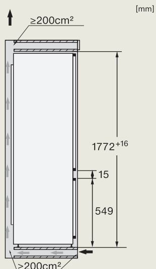
KF 7742 D
