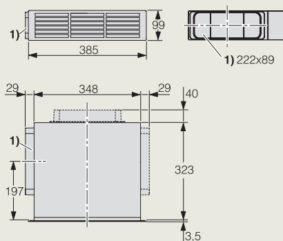
DUU 1000-2 Ombouwset voor luchtcirculatie
