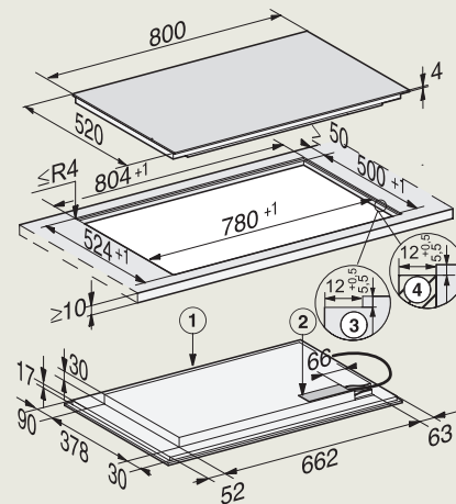
KM 7576 FL (vlakbouw)
