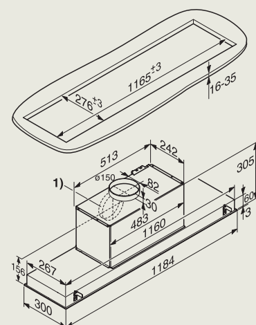
DA 2628 inbouwgroep
