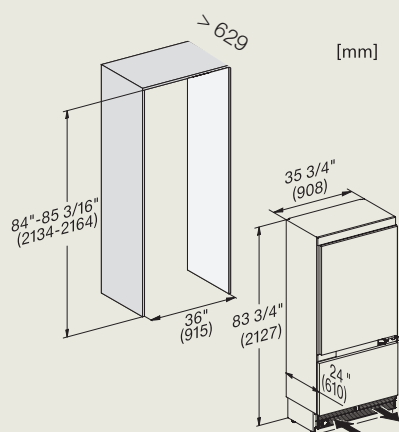
KF 2902 Vi
