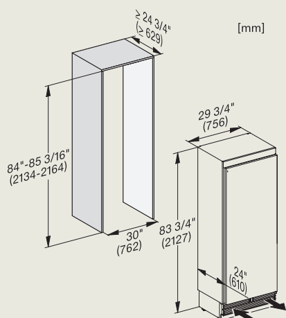
K 2802 Vi
