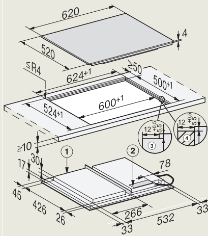
KM 7667 FL (vlakbouw)
