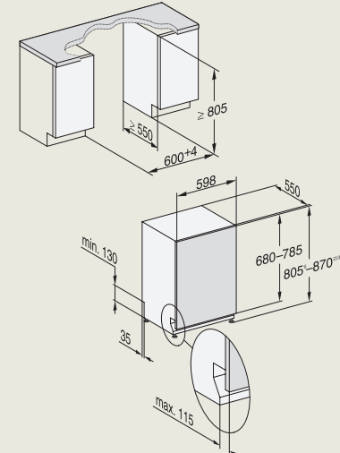
G 7000 volledig integreerbare vaatwassers 60 cm FrontFit
