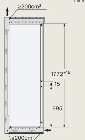
KFN 7744 D, KFN 7744 C, KFN 7764 C, KFN 7785 C
