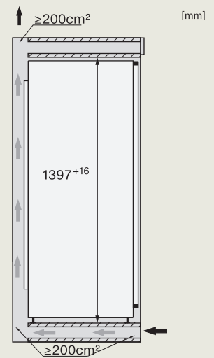
FNS 7470 D
