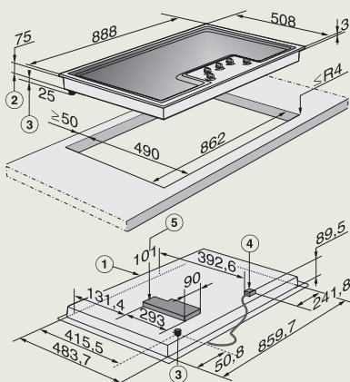
KM 2356-1
