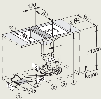
CSDA 7001 FL (opbouw)
