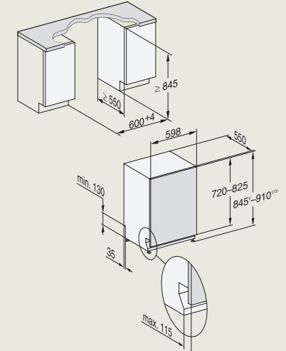
G 7000 volledig integreerbare vaatwassers 60 cm XXL FrontFit
