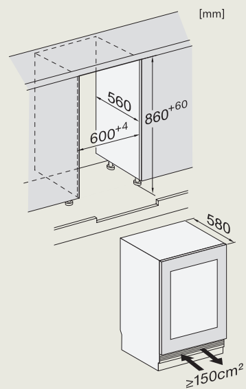
KWTUS 7196 E
