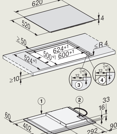
KM 7363 FL
