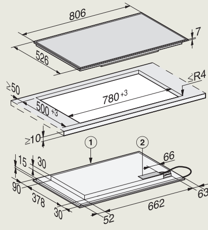
KM 7575 FR
