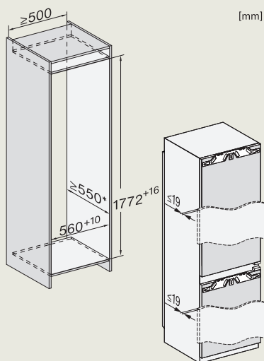
KF 7742 D
