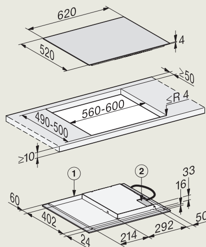
KM 7361 FL
