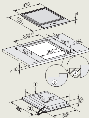
CS 7632 FL TeppanYaki (vlakbouw)
