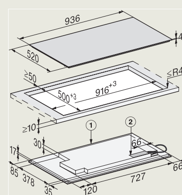
KM 7899 FL (opbouw)
