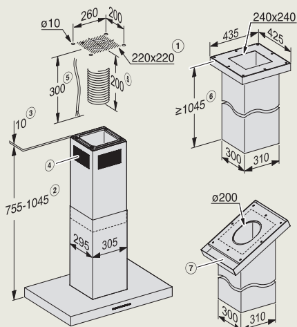
DA 4208 D, DA 4248 V D eilanddampkappen
