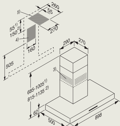
DA 4298 W (EXTERN) wanddampkap
