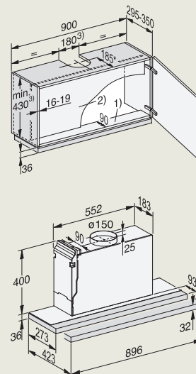
DAS 2920, DAS 4920
