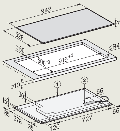
KM 7699 FR
