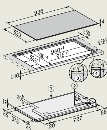
KM 7899 FL (vlakbouw)
